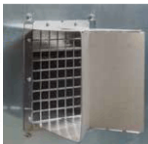
воздухораспределительная камера с двумя выходами (левый и правый)
